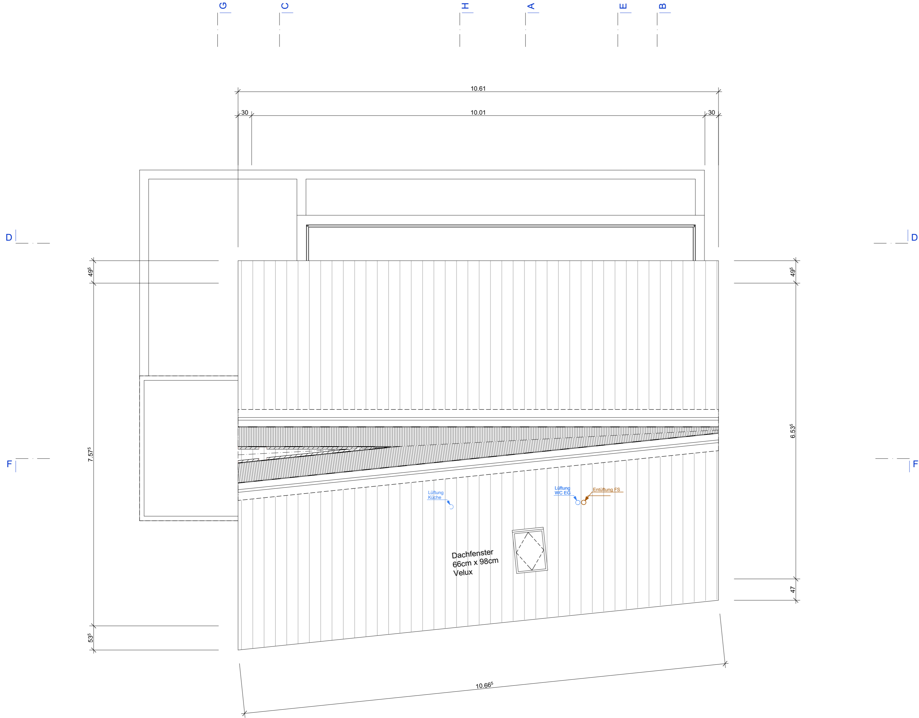
DACHANSICHT
